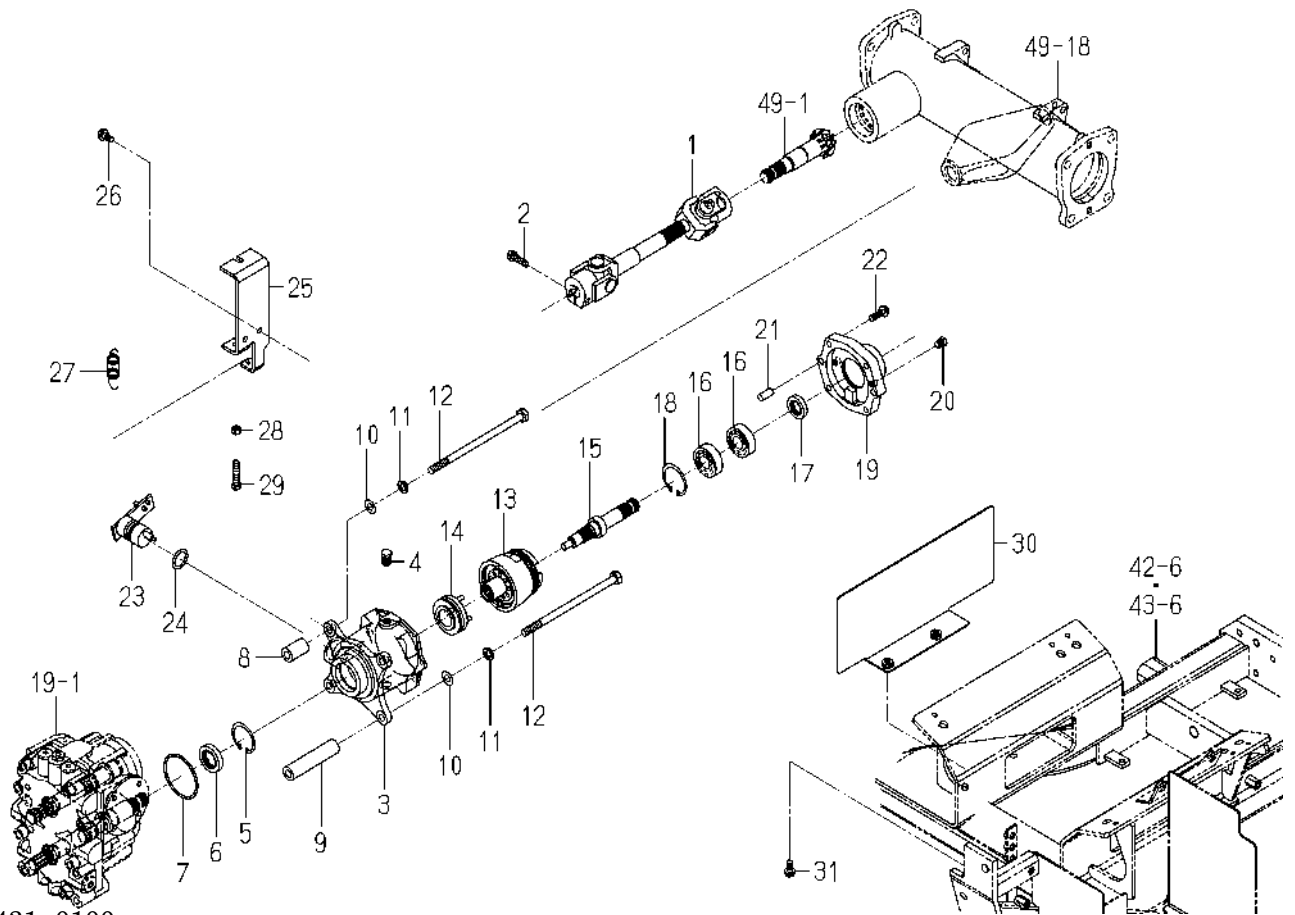
FIG. 48 AUTO(4WD)SYSTEM
