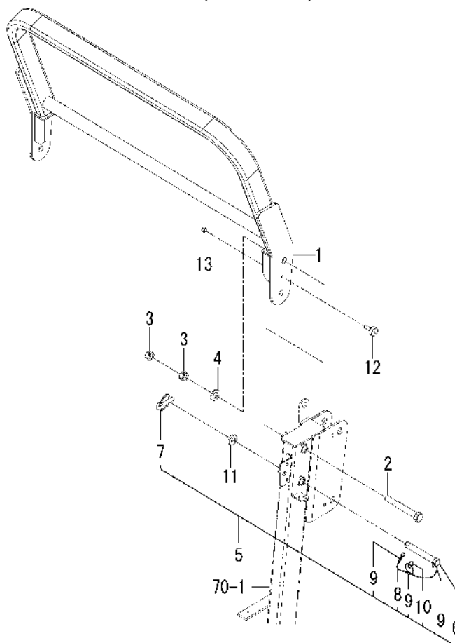
FIG. 71 FRAME(UPPER)SYSTEM
