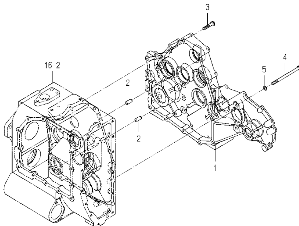
FIG. 17 METAL(HST)SYSTEM
