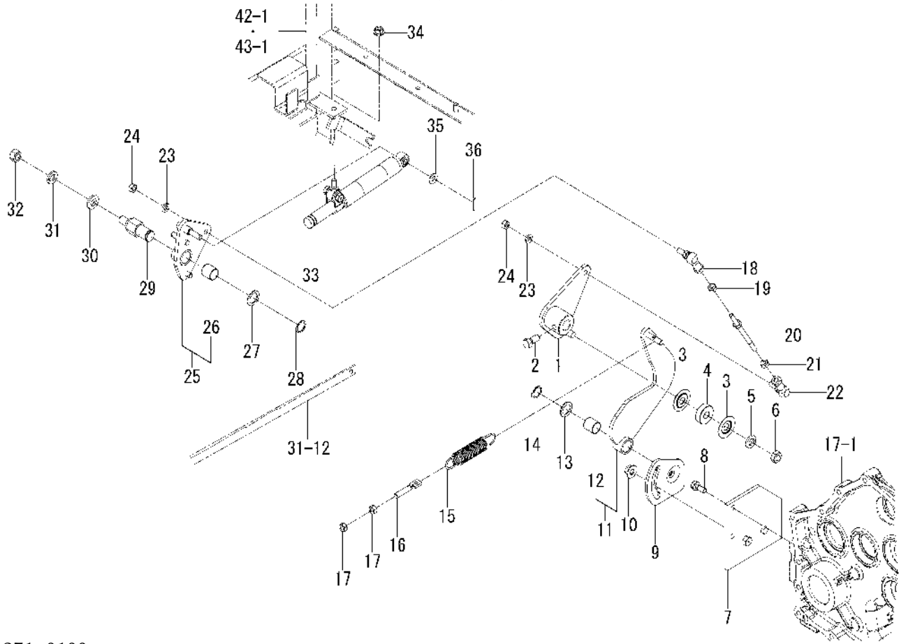
FIG. 30 LINK(HST)SYSTEM
