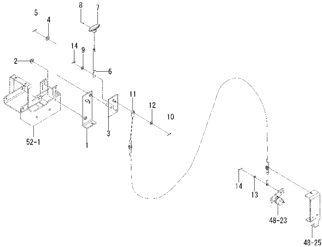
FIG. 47 LEVER(4WD)SYSTEM
