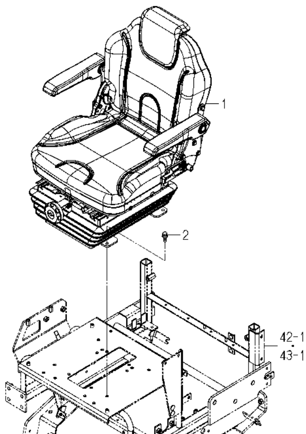
FIG. 61 SEAT SYSTEM(Z TYPE-STANDARD/ EXCEPT Z TYPE-OPTION)
