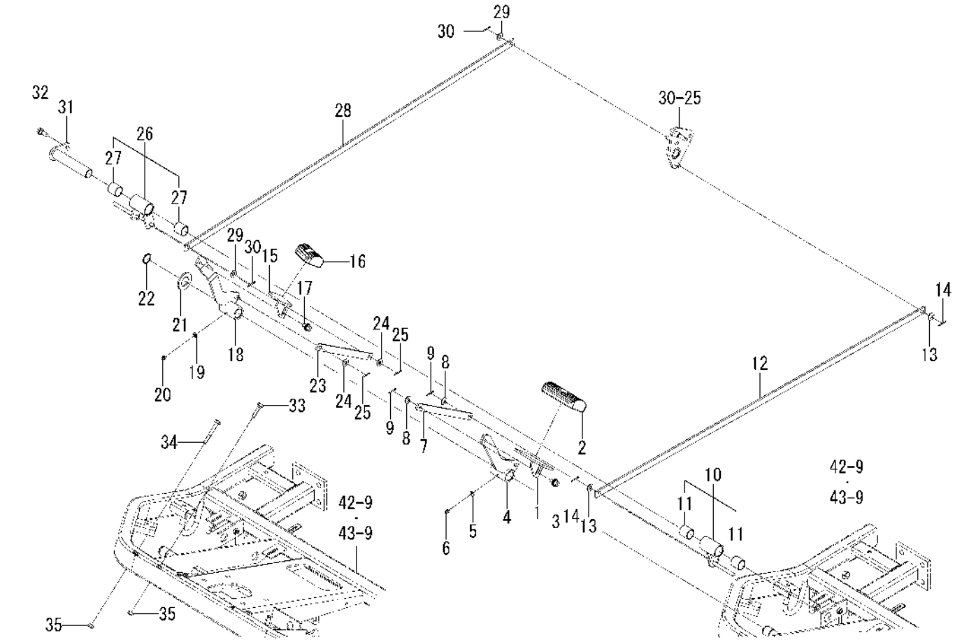
FIG. 31 PEDAL(HST)SYSTEM
